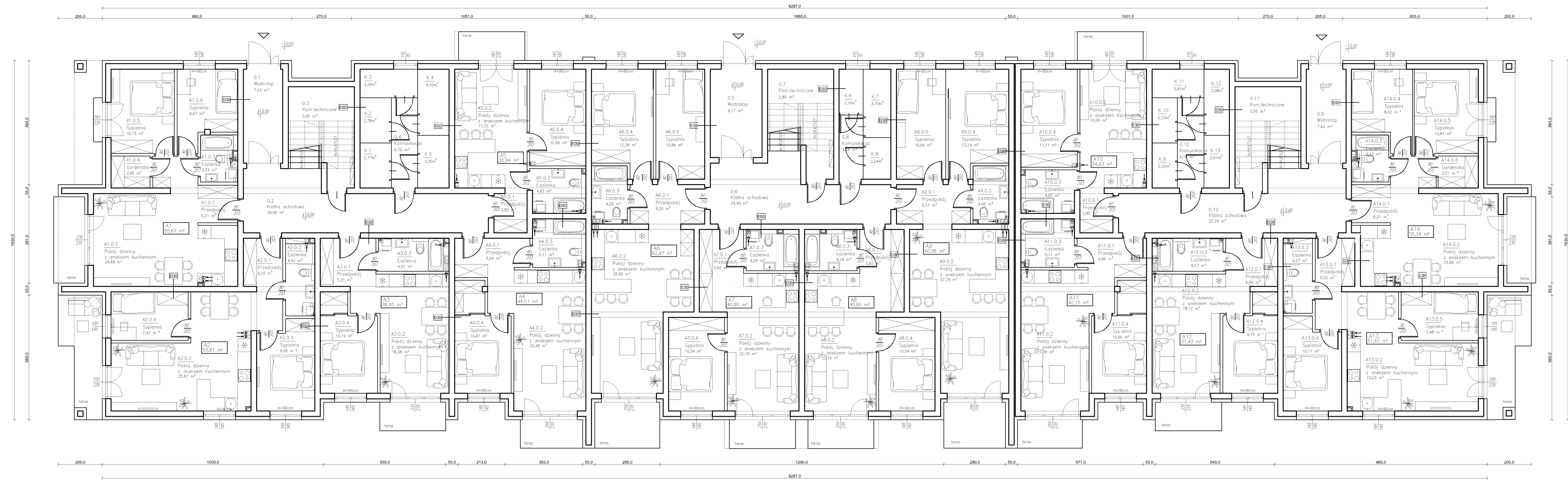
RZUT PARTERU
