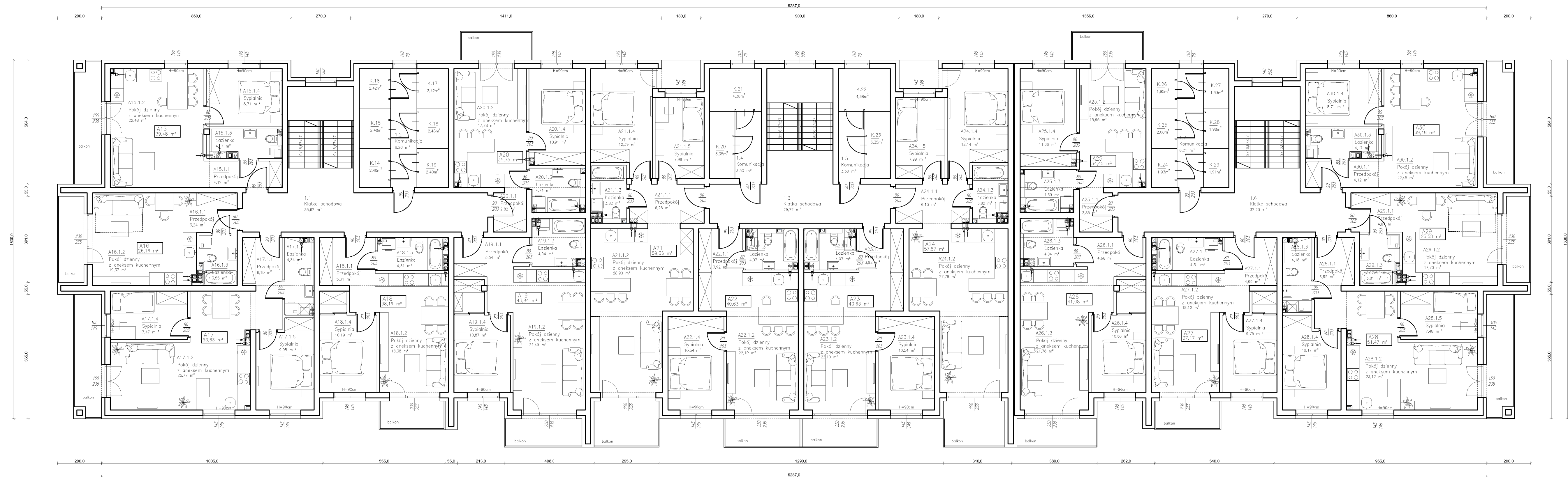
RZUT PIĘTRA
