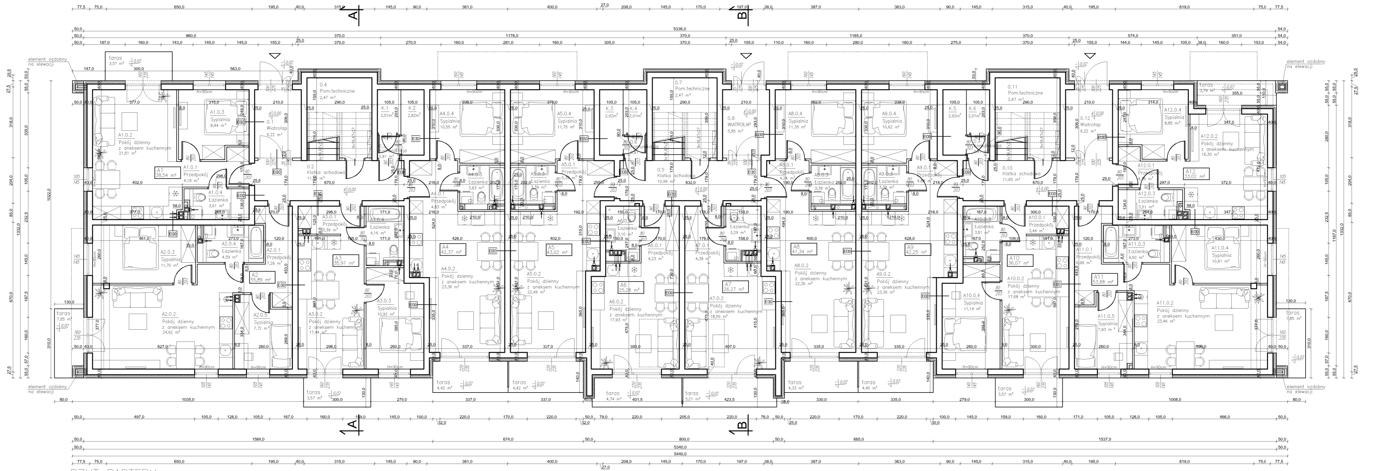
RZUT PARTERU
